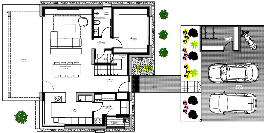
PLANTA BAJA ESCALA 1/200
